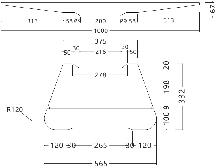
剖视图
