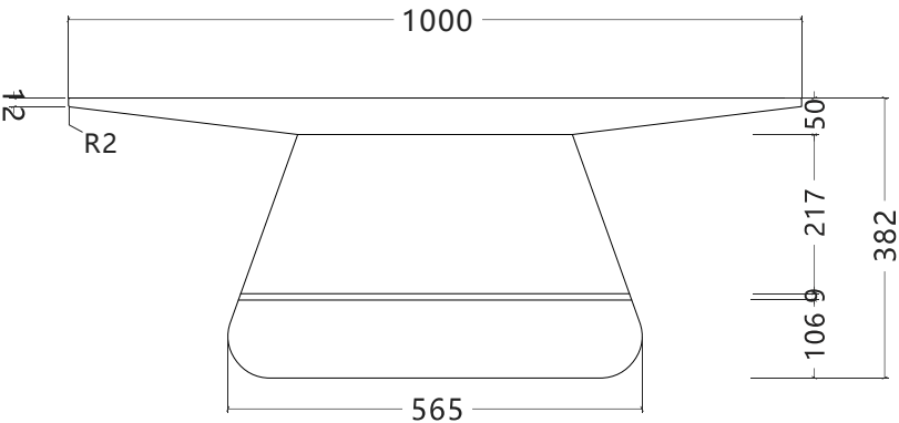
正视图
